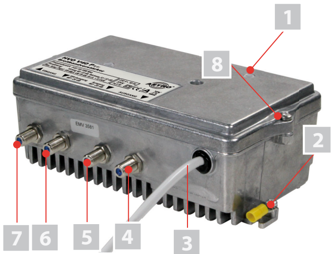
Bild 1: Verstärker HVO V40 P
