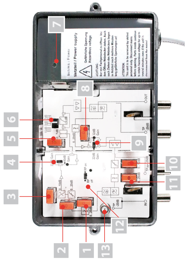
Bild 2: Verstärker HVO V40 P, Innenansicht
