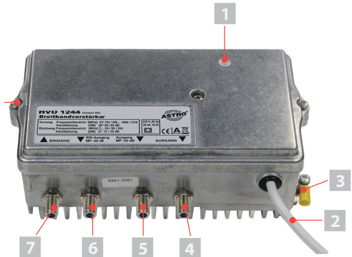
Bild 1: Verstärker HVO 1244
