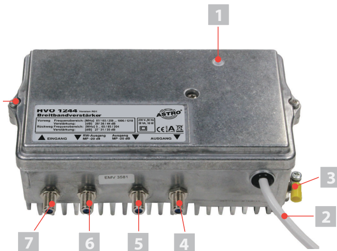
Bild 1: Verstärker HVO 1244
