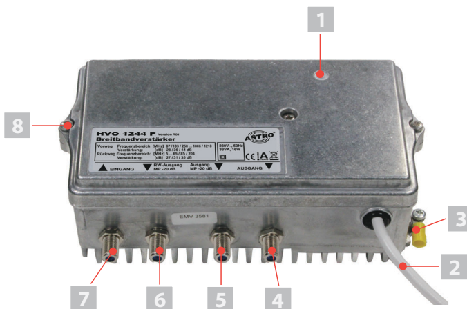
Bild 1: Verstärker HVO 1244 P
