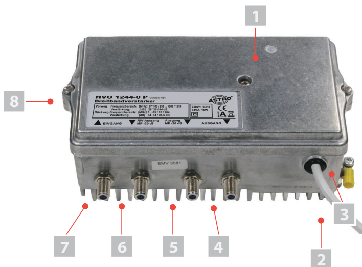
Bild 1: Verstärker HVO 1244-0 P
