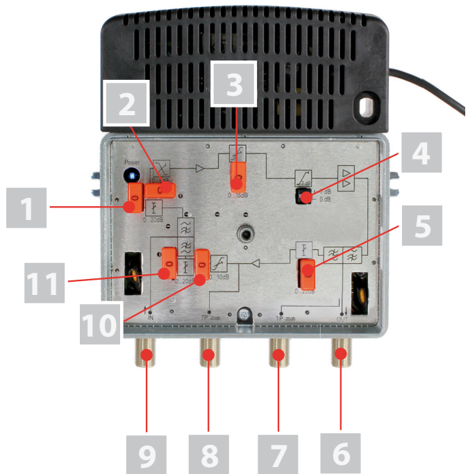
Bild 2: Verstärker HV 536, Innenansicht
