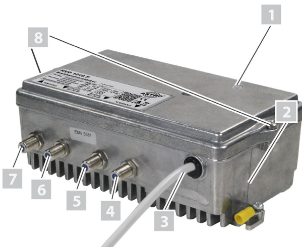
Bild 1: Verstärker HVO 1218 P
