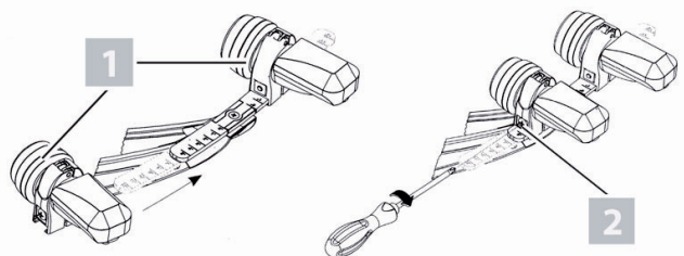
Bild 4: Speiseeinheiten an der Multifeedplatte montieren
