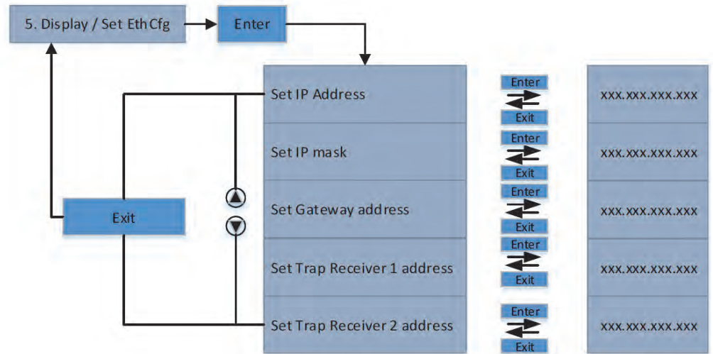
Figure 6: „Display / Set Ethernet“ menu
