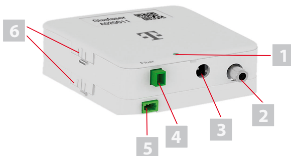
Bild 2: OFN46-WDx-ALC komplett
